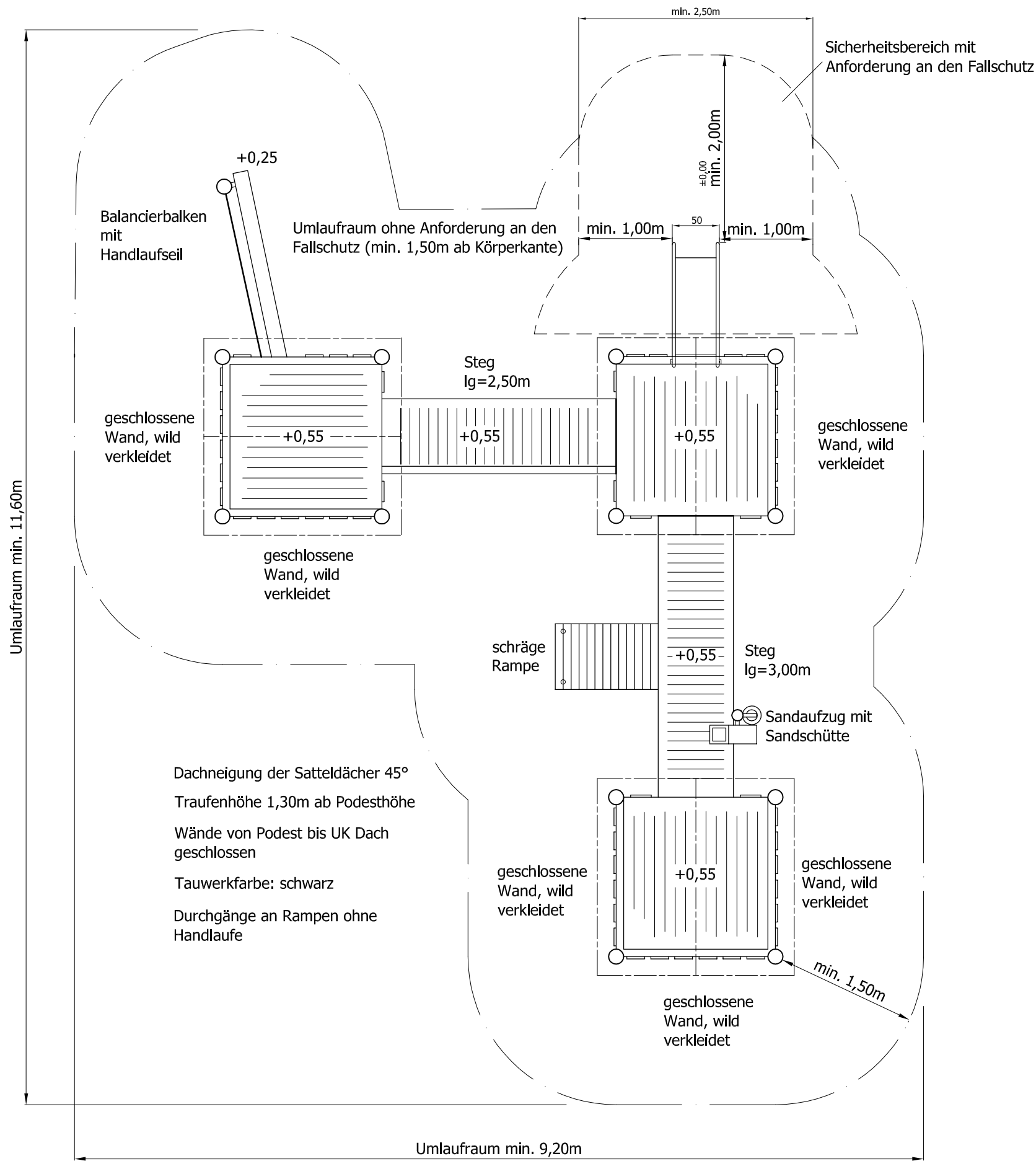
Draufsicht -1:50-
