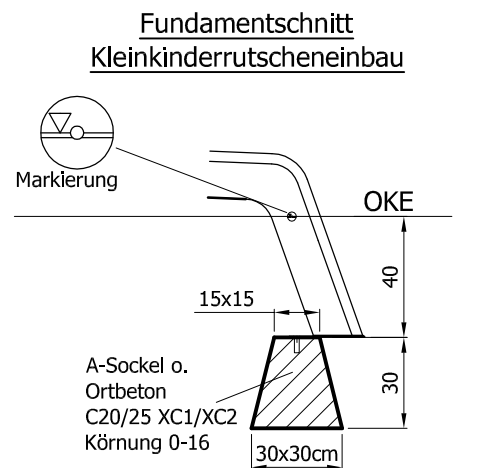
M -1:25-
